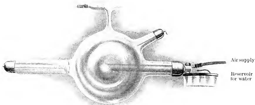
FIG. 216.—Dessaeur therapeutic tube.
